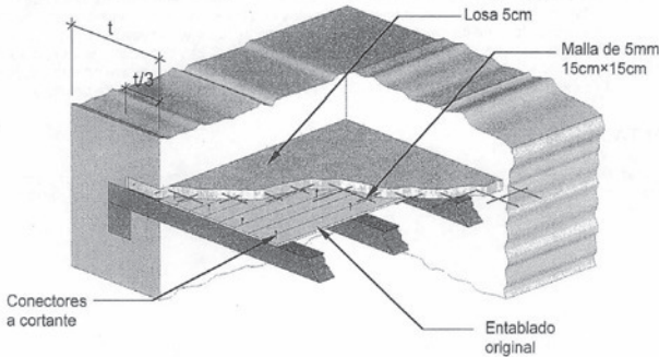
Figura 7.3.1-1. Reforzamiento de diafragma mediante construcción de plaqueta de concreto
