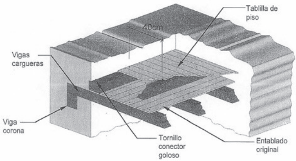
Figura 7.3.2-1. Reforzamiento de diafragma mediante entablado complementario
