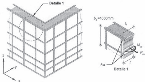
Figura 8.6.1-1. Flexión con respecto al eje vertical combinada con fuerza axial horizontal
