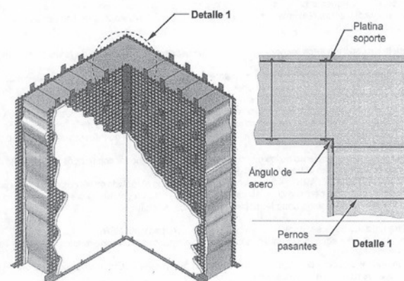
Figura 7.2.3-1. Sistema de reforzamiento con mallas de acero o sintéticas
