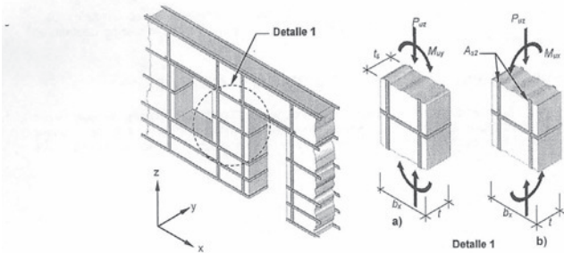
Figura 8.5-1. Flexión con respecto al eje horizontal combinada con fuerza axial vertical
