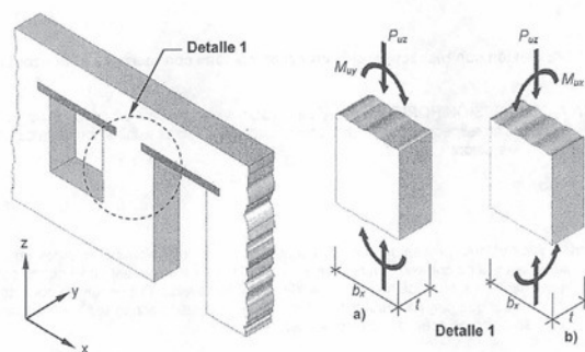
Figura 6.5.1-1. Flexión con respecto al eje horizontal combinada con fuerza axial vertical
