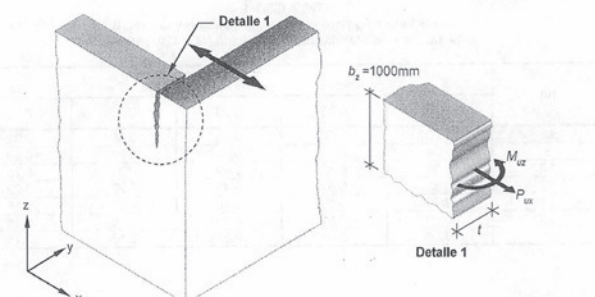
Figura 6.6.1-1. Flexión con respecto al eje vertical combinada con fuerza axial horizontal
