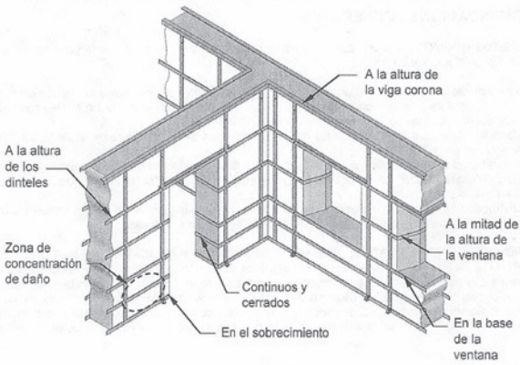
Figura 7.2.1-1. Sistema de reforzamiento con entramados de madera, acero, plástico o similar.
